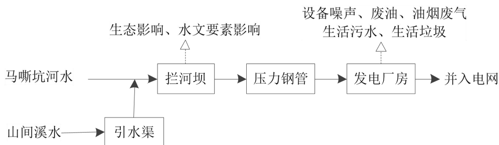
图 2.4-1 工艺流程及产污节点图
