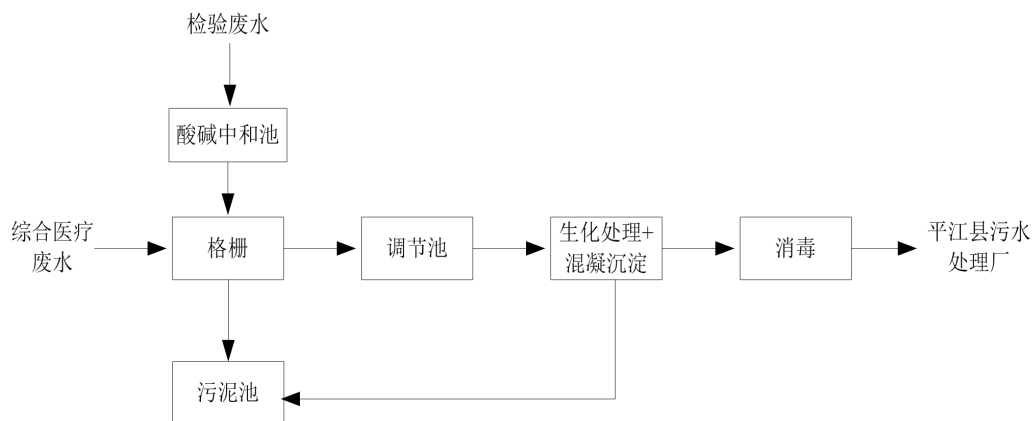
图 4-1 医院废水处理站工艺流程图
