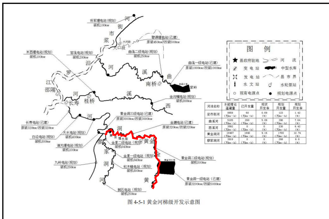
图 2-1 黄金洞河水系梯级开发现状
