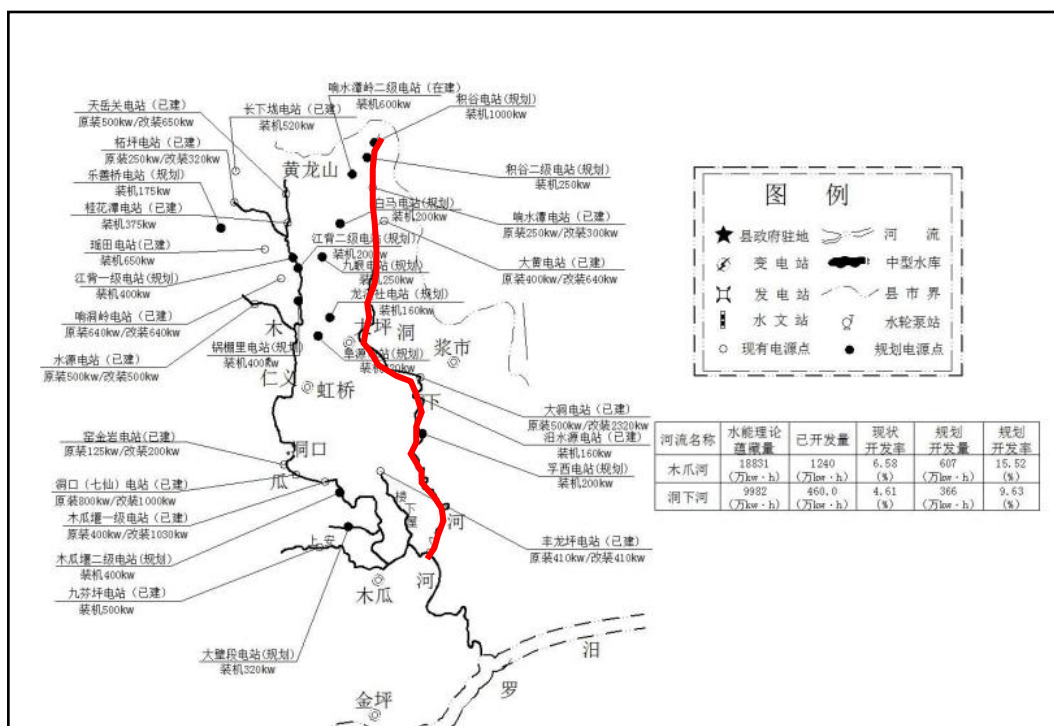
图 2-1 洞下河水系梯级开发现状
